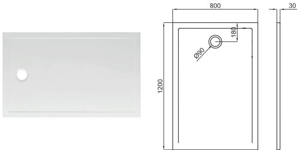
120x80 ceramic shower tray Receveur de douche 120x80 ceramique
