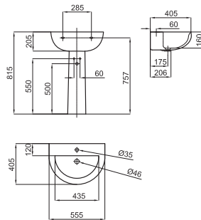
CITY N. 55 cm. wall hung basin with overflow and fixing kit 100041225 - N421040000. Lavabo 55 cm. avec trop plein et fixations 100041225 - N421040000.
