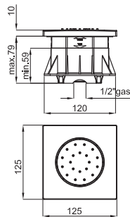
1/2" concealed body jet. Minimum flow rate required: 3,55 l/min. at 3 bar Buse latérale douche 1/2". Requiert un débit minimum à 3 bars de 3,55 l/min.
