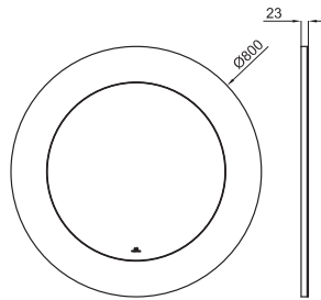
Ø80 cm. Round mirror. Dark colour frame. Black lacquered wood on the back. Miroir circulaire de Ø80 cm. Encadrement miroir sombre et bord en bois laqué noir.
