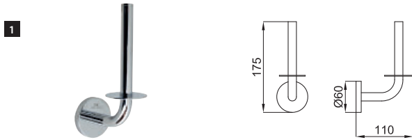
1 Spare roll holder Porte-papier de réserve
