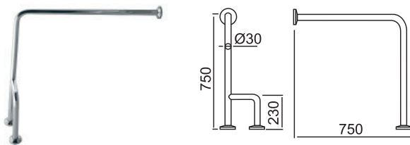
Grab rail 3 wall-floor Barre de maintien fixation sol-mur
