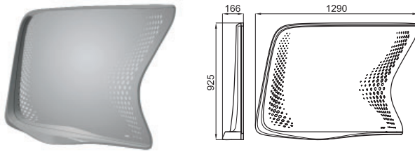
MIRROR WITH LED LIGHT for LEFT bowl basin Miroir avec lumière pour lavabo gauche
