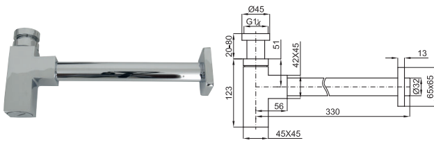
1 ACRO - Bottle trap ACRO - Siphon bouteille lavabo
